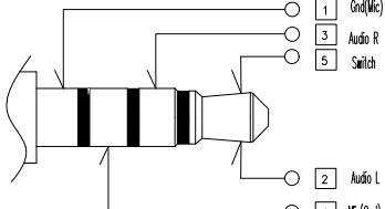
SCHEMATIC(PLUG IN)
